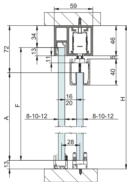
STAR XL + VIDRIO FIJO | FIXED GLASS | VERRE FIXE
