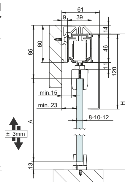
EXCELLENCE XL + SEPARADOR | SEPARATOR | SÉPARATEUR A= H-85
