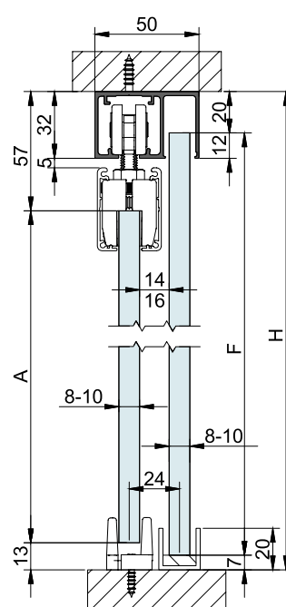
STAR VIDRIO FIJO | FIXED GLASS | VERRE FIXE
