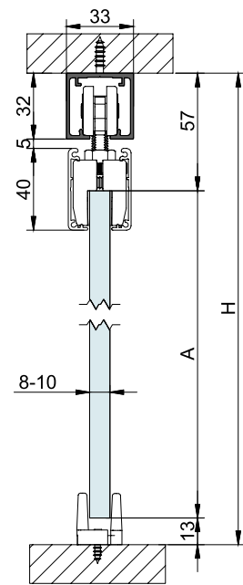
STAR A= H-70
