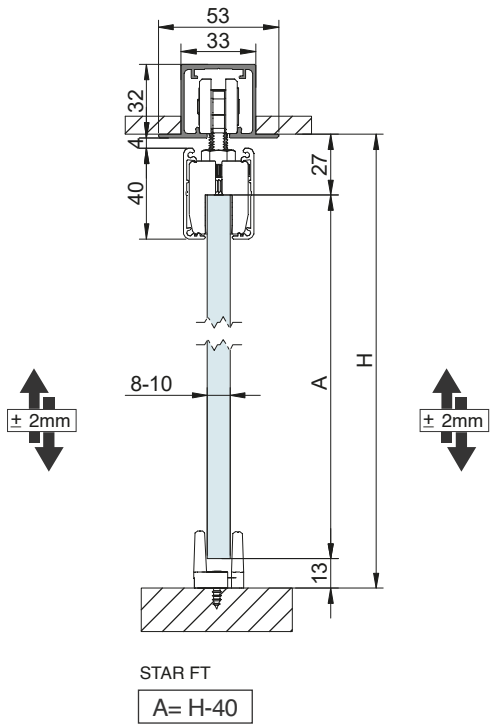
STAR FT VIDRIO FIJO
