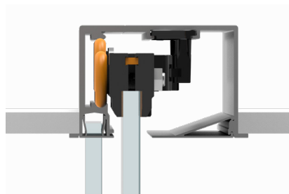
FALSO TECHO CON VIDRIO FIJO
