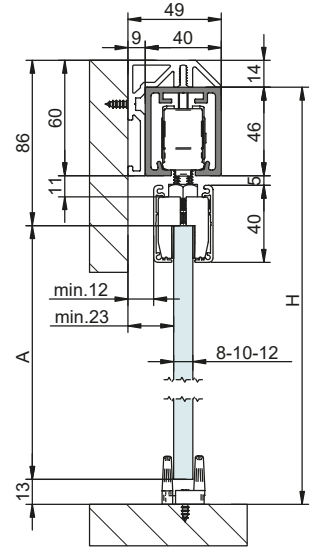
STAR XL + SEPARADOR | SEPARATOR | SÉPARATEUR A= H-85 F= H-47
