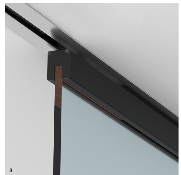
A Perfil funda FT XL | Support FT XL track | Rail de couverture FT XL. B Perfil Star XL | Star XL track | Rail Star XL. C Diseño de perfil con avellanado integrado | Track design with drilled countersink | Conception de rail avec fraisage intégré.
