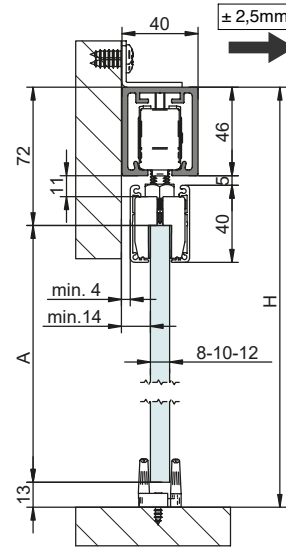
STAR XL A= H-85 F= H-47
