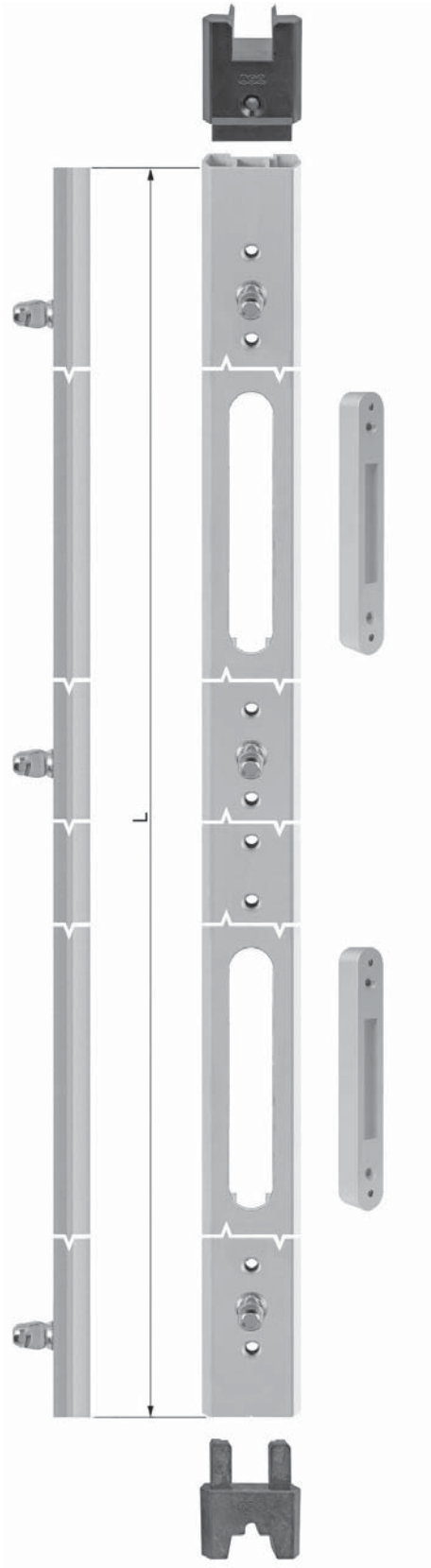
Perfil de cierre POSEIDON para hojas coaxiales con tapa
