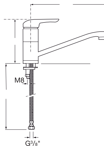
Dibujo técnico
