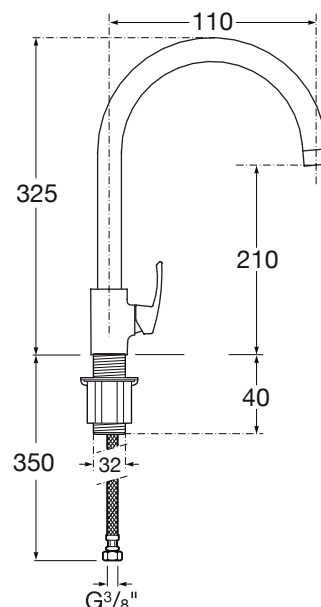
Dibujo técnico
